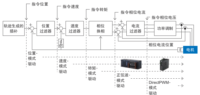
可编程多轴 运动控制器 CK3M
