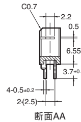
断面AA
