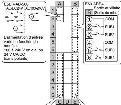
E5ER-Q4B
