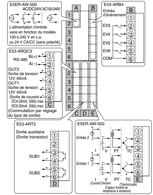
E5ER-QT3DW-FLK (Type à 2 entrées)
