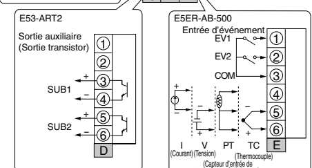
E5ER-QT3DW-FLK (Type à 2 entrées)
