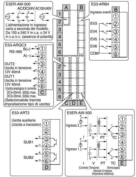
E5ER-QT3DW-FLK (Tipo a 2 ingressi)
