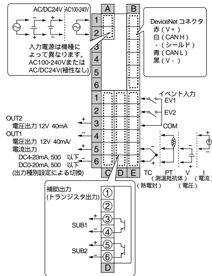
E5ER-QTB-DRT
