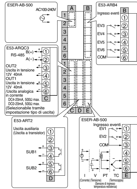
E5ER-QT3DB-FLK
