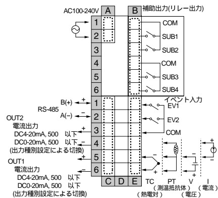
E5ER-C43B-FLK
