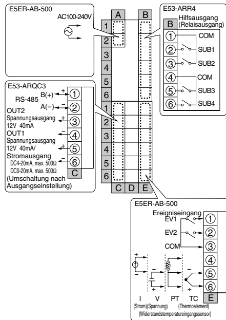
E5ER-Q43B-FLK
