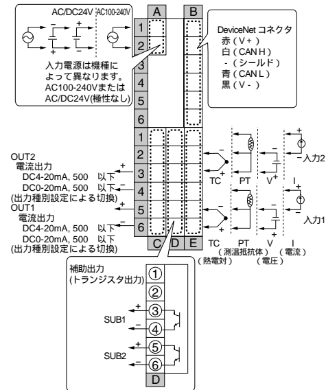
E5ER-CTW-DRT(2入力タイプ)
