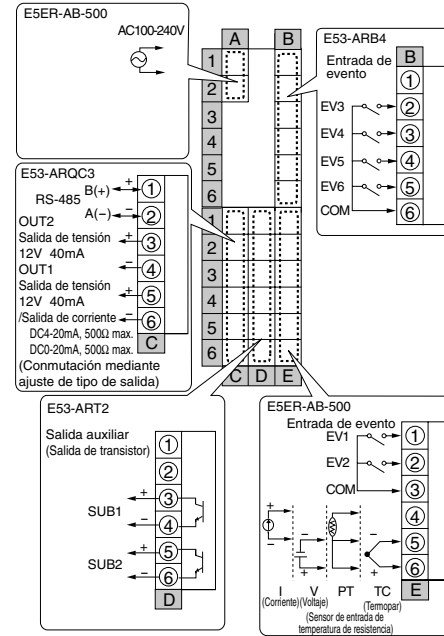
E5ER-QT3DB-FLK
