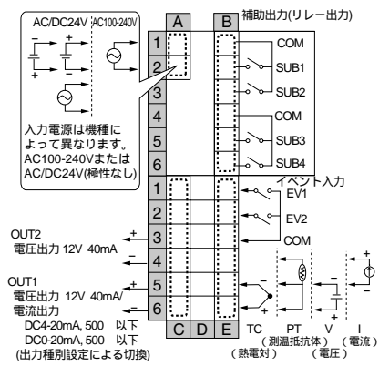
E5ER-Q4B
