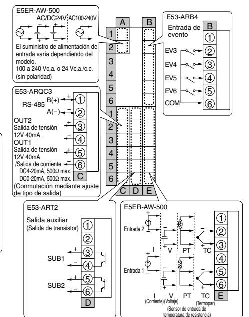
E5ER-QT3DW-FLK (tipo 2 entradas)
