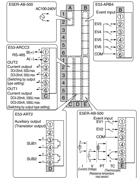
E5ER-CT3DB-FLK
