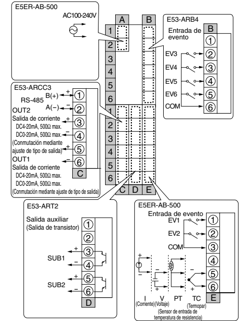
E5ER-CT3DB-FLK
