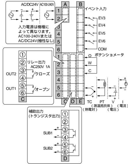
E5ER-QTB-DRT
