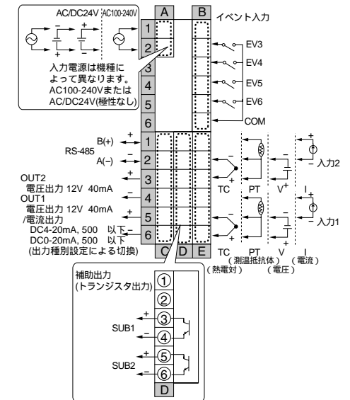
E5ER-QT3DW-FLK
