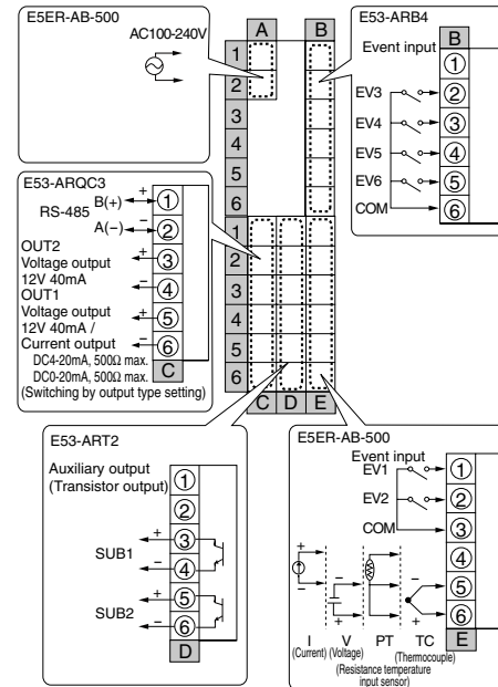
E5ER-QT3DB-FLK
