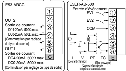
E5ER-C43B-FLK
