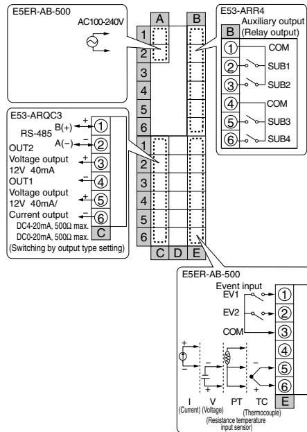
E5ER-Q43B-FLK
