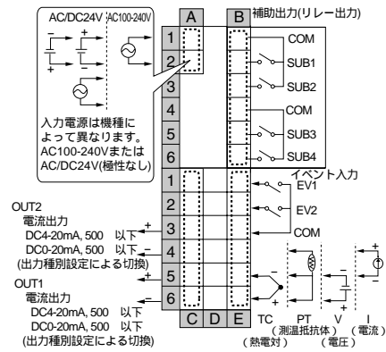
E5ER-C4B
