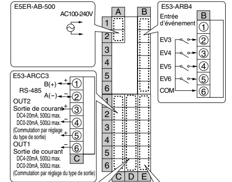
E5ER-CT3DB-FLK
