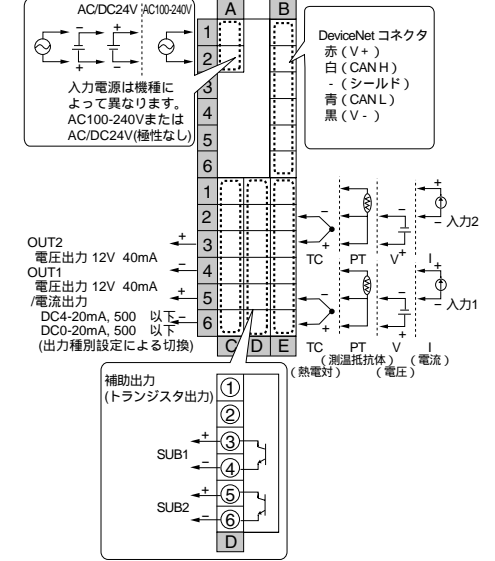
E5ER-QTW-DRT(2入力タイプ)
