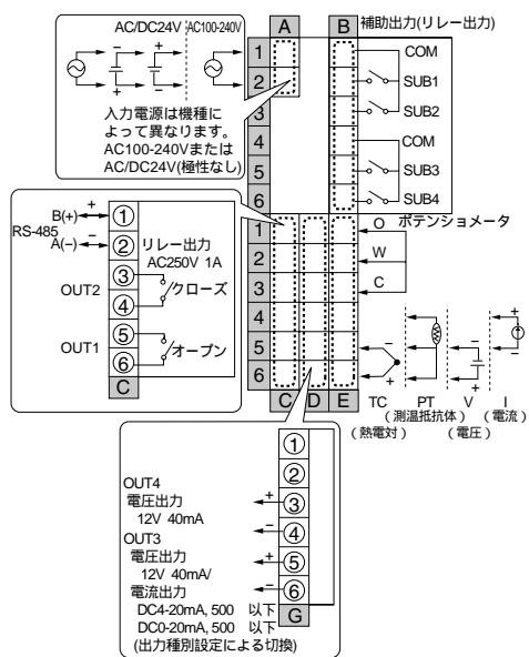
E5ER-PRQ43F-FLK
