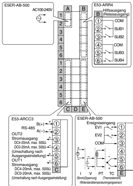
E5ER-C43B-FLK
