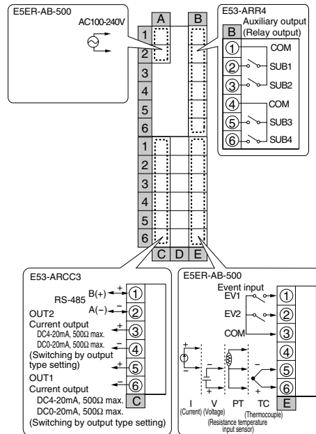
E5ER-C43B-FLK
