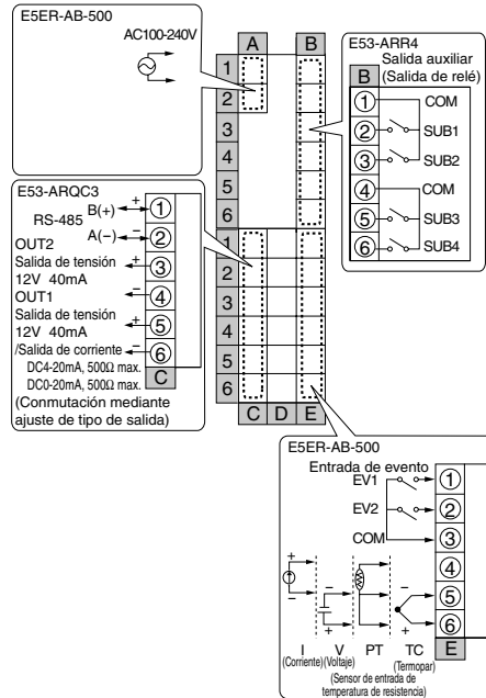
E5ER-Q43B-FLK
