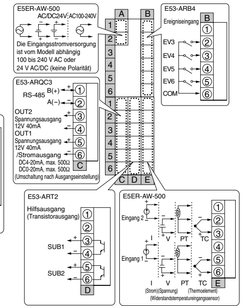
E5ER-QT3DW-FLK (Ausführung mit 2 Eingängen)
