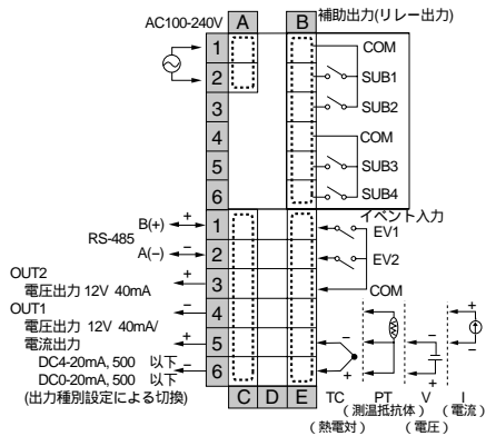
E5ER-Q43B-FLK
