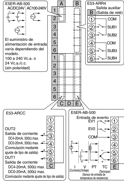
E5ER-C4B
